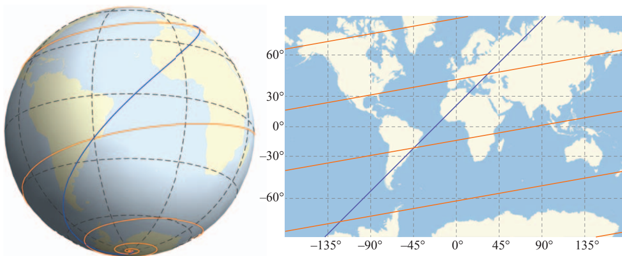
Figura 1.41: Linhas de rumo (loxodromia) em uma esfera (esquerda) convergem para os polos (exceto as linhas com inclinação zero, i.e., ao longo das latitudes). A linha azul faz um ângulo constante de 45^\circ com os meridianos; a linha laranja tem um ângulo de 80^\circ (a partir do Norte, em sentido horário). Na projeção de Mercator (direita, limitado aqui entre as latitudes \pm 75^\circ ), as loxodromias são linhas retas. Note que as linhas de rumo geralmente não correspondem às distâncias mais curtas entre dois pontos na superfície da esfera (a distância mais curta é a geodésica).
