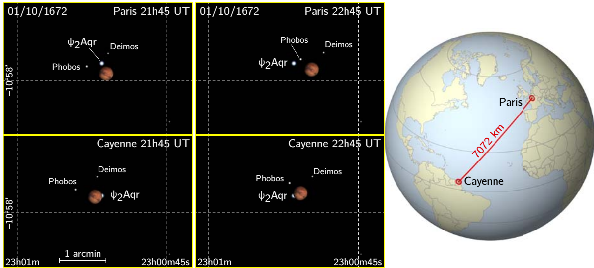
Figura 4.44: Esquerda: Simulação da observação do início e fim da ocultação de \psi_2 Aqr por Marte. A paralaxe de Marte foi obtida com as medidas de Giovanni Cassini em Paris e Jean Richer na Guiana Francesa. Em Cayenne, foi observada a ocultação da estrela \psi_2 Aqr por Marte, enquanto que, em Paris, Marte passa a alguns segundos de arco da estrela. Apesar de Phobos e Deimos estarem representados nesta figura, eles só foram descobertos em agosto/1877 por Asaph Hall. Direita: Ilustração da distância entre Cayenne e Paris que serviu de base para a medida da paralaxe diária de Marte.
