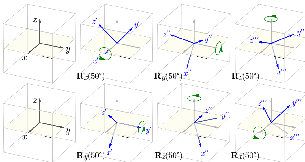
Figura 1.37: Não comutatividade das rotações: a ordem dos fatores altera o resultado final. Acima: Rotação \mathbf{R}_x, \mathbf{R}_y, \mathbf{R}_z , cada uma com 50^\circ , operando sucessivamente nos vetores (x, y, z) \rightarrow (x', y', z') \rightarrow , etc. Abaixo: Rotação \mathbf{R}_y, \mathbf{R}_z, \mathbf{R}_x , cada uma com 50^\circ . A orientação dos eixos nos painéis finais, acima e abaixo, (x''', y''', z''') são claramente diferentes.
