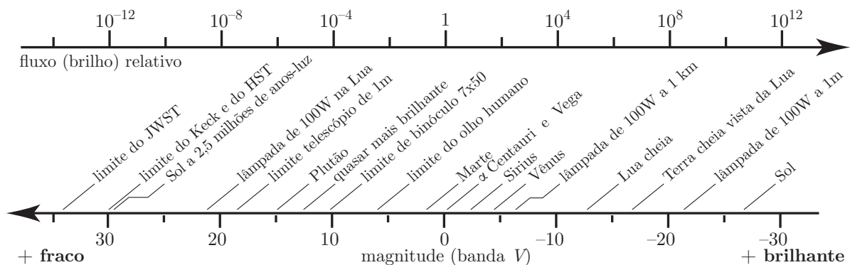
Figura 1.2: Escala de magnitude na banda visível (grosseiramente, é a faixa de luz que observamos a olho nu) com alguns exemplos representativos. Keck é um telescópio de 10 metros de diâmetro no Havai, HST é o telescópio espacial Hubble. A magnitude dos planetas corresponde à condição mais favorável. Vega, Sirius e \alpha Centauri estão entre as estrelas mais brilhantes vistas da Terra.
