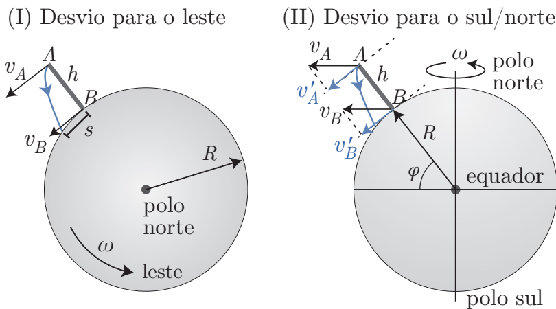
Figura 2.14: (I) objeto lançado de uma torre de altura h não cai verticalmente, mas sobre um desvio para o Leste (trajetória azul) (II) No Hemisfério Norte, o corpo também sofre um desvio para o Sul (e vice-versa no Hemisfério Sul). A velocidade angular da Terra no equador é \omega = 2\pi/P , P é o período de rotação.
