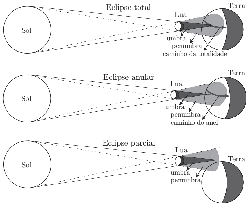
Figura 4.22: Representação dos eclipses total, anular e parcial do Sol. Para observadores que se encontram na umbra, o disco solar está completamente oculto pela Lua. Para os observadores que se encontram na penumbra, o disco solar está apenas parcialmente oculto (para este observador é um eclipse parcial). Caso a Terra estivesse mais próxima do Sol ou a Lua mais distante da Terra, o eclipse seria anular (o disco aparente da Lua seria menor que o disco solar). No caso do alinhamento Sol-Lua não ter intersecção com o disco da Terra, temos um eclipse não-central que será observado apenas como parcial (a não ser em casos muito raros, onde o eclipse não-central é total ou anular). A seta indica o movimento da sombra na superfície da Terra (de Oeste para Leste).
