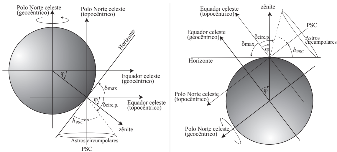
Figura 1.30: Geometria correspondente à declinação máxima de astros visíveis e de astros circumpolares para um observador no Hemisfério Sul. Esquerda: Perspectiva onde o equador está na horizontal (apropriado para coordenadas equatoriais). Direita: perspectiva onde o horizonte do observador está na horizontal (apropriado para coordenadas horizontais).
