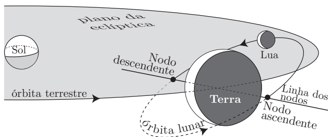
Figura 4.28: Geometria da órbita da Lua em relação à eclíptica. As órbitas não são coplanares e a reta da intersecção é chamada linha dos nodos onde se encontram os nodos ascendente e descendente. A inclinação da órbita da Lua em relação à eclíptica é de cerca de 5^{\circ}1' .
