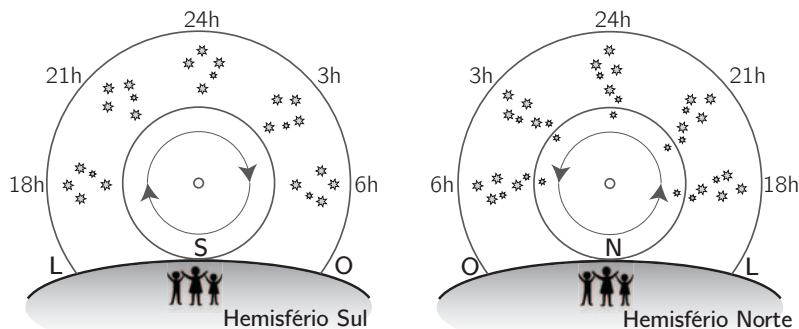
Figura 1.29: Esquerda: Observação do movimento diário dos astros no Hemisfério Sul no sentido horário. Direita: No Hemisfério Norte, os astros têm um movimento aparente anti-horário, quando olhamos na direção do Norte geográfico
