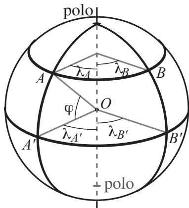
Figura 1.40: Comprimento de segmentos de arco. O segmento \widehat{A'B'} faz parte do círculo principal (equador), o segmento \widehat{AB} , do pequeno círculo de latitude \varphi .
