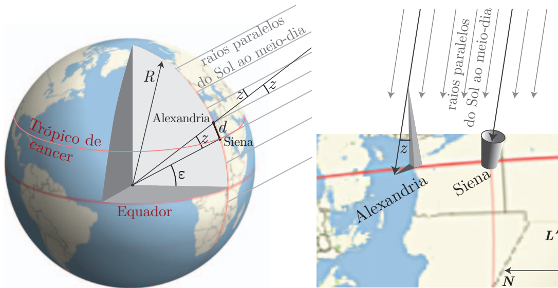
Figura 4.36: Ao meio-dia do solstício de Verão no Hemisfério Norte, o Sol tem um ângulo zenital z em Alexandria e zero em Siena (hoje, Assuã). A distância entre as duas cidades é d , R é o raio da Terra e \varepsilon é a obliquidade da eclíptica na época de Eratóstenes. Note que o ângulo zenital z é igual à diferença entre as latitudes de Alexandria e Assuã.
