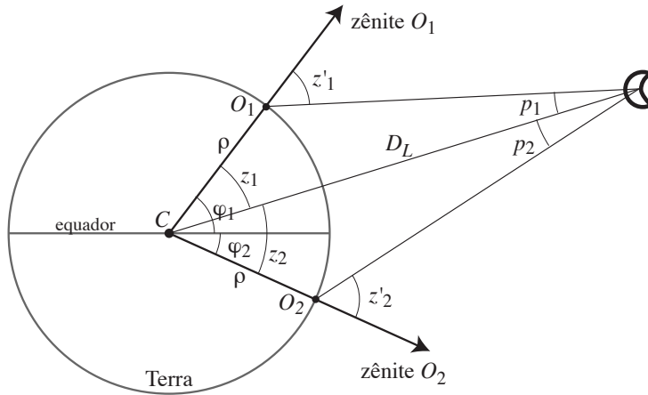
Figura 4.39: Medidas simultâneas da paralaxe diária da Lua por dois observadores, O_1 e O_2 , no mesmo meridiano. O raio da Terra é \rho e D_L é a distância geocêntrica da Lua.
