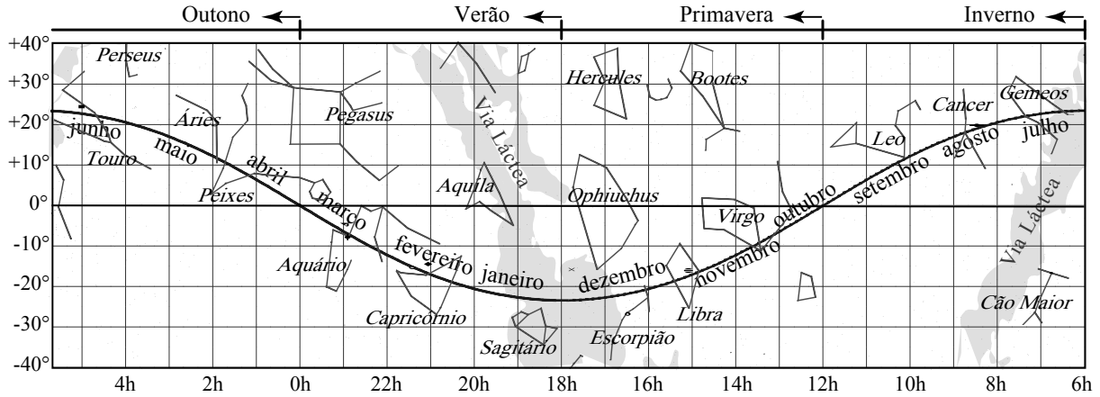
Figura 1.25: Detalhe da esfera celeste em coordenadas equatoriais mostrando a eclíptica com os meses que correspondem à posição do Sol. O início das estações para o Hemisfério Sul está assinalado acima da figura. As constelações do Zodíaco (e Ophiucus) estão no caminho aparente do Sol, com declinação entre \pm 23^{\circ}44' .
