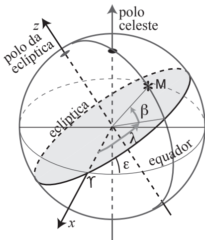
Figura 1.22: Sistema de coordenadas eclípticas. O astro M tem coordenadas longitude eclíptica ( \lambda ) e latitude ( \beta ). A inclinação da eclíptica em relação ao equador celeste é \varepsilon que vale aproximadamente 23^{\circ}26'21'' atualmente.
