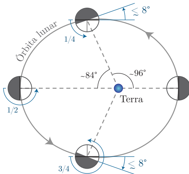
Figura 4.35: Libração geométrica (óptica) em longitude. O observador hipotético está no polo Norte da órbita lunar. A Lua é mostrada em intervalos de tempo iguais, de um quarto de rotação. A trajetória percorrida na órbita é diferente, de acordo com a 2ª lei de Kepler. O semi-disco cinza escuro representa a face oculta da Lua (não tem nada a ver com face iluminada). O ângulo de libração em longitude representado aqui é um valor máximo, quando se leva em conta a perturbação do Sol na órbita da Lua.
