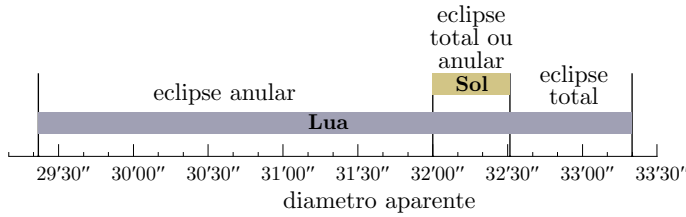
Figura 4.23: Comparação dos diâmetros aparentes do Sol e da Lua. A variação ocorre devido à elipticidade (achatamento) das órbitas da Terra e da Lua. Como a órbita lunar é mais excêntrica, a variação do tamanho aparente é maior.
