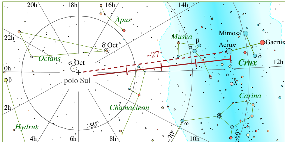
Figura 1.9: O Cruzeiro do Sul pode ser usado para localizar o polo Sul celeste e o polo Sul geográfico. A linha tracejada indica a prolongação aproximada do Cruzeiro até o polo celeste, \sim 27^\circ , cerca de 4 vezes o eixo maior da cruz. Também estão destacadas duas estrelas próximas do polo, que podem ser usadas como referência: delta e sigma Octans. A Via Láctea está representada em tons de azul.
