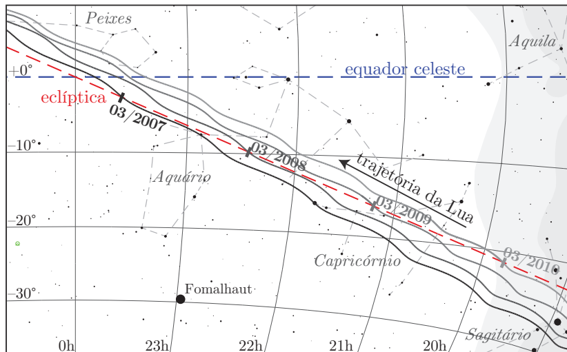
Figura 1.12: A órbita lunar é exibida em 4 momentos (linhas cinzas) separados por aproximadamente um ano cada um. A linha vermelha tracejada representa a eclíptica e a linha azul o equador celeste. Podemos ver que o nodo da órbita retrocede, isto é, se movimenta no sentido oposto à Lua em sua órbita. Note também a inclinação da órbita lunar em relação à eclíptica.
