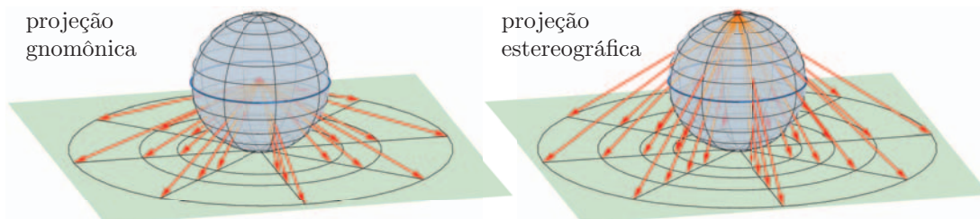
Figura 1.43: Na projeção gnomônica os raios emanam do centro da esfera; na projeção estereográfica os raios vêm do polo oposto ao plano onde a esfera é projetada. Em ambos os casos deste exemplo o aspecto é polar. Para a projeção ortográfica, quando os raios são paralelos e vêm do infinito, veja a Fig. 1.42.
