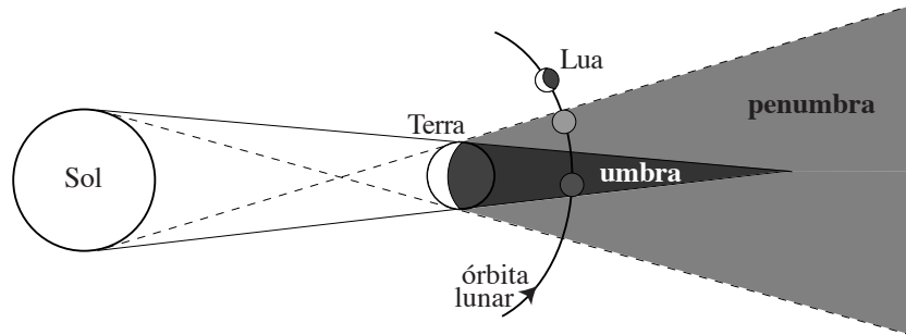
Figura 4.26: Representação de um eclipse da Lua ao passar pela sombra da Terra.
