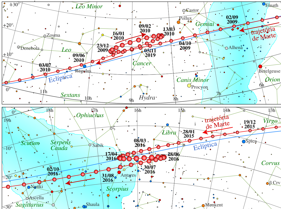
Figura 1.14: Dois exemplos do movimento aparente de Marte na esfera celeste ilustrando o movimento retrógrado. O intervalo entre duas posições ao longo da trajetória corresponde a 8 dias. O tamanho aparente de Marte está representado de forma aproximada (e fora de escala). O movimento retrógrado dos planetas externos ocorre quando o planeta passa pela oposição, por isto o tamanho aparente aumenta (Fig 4.14 na seção 4.9). Também estão indicados algumas estrelas brilhantes, constelações e as coordenadas equatoriais. A Eclíptica está representada pela linha azul. Podemos notar que a trajetória de Marte é próxima, mas não é exatamente sobre a eclíptica devido à inclinação relativa do seu plano orbital em relação ao plano orbital da Terra.
