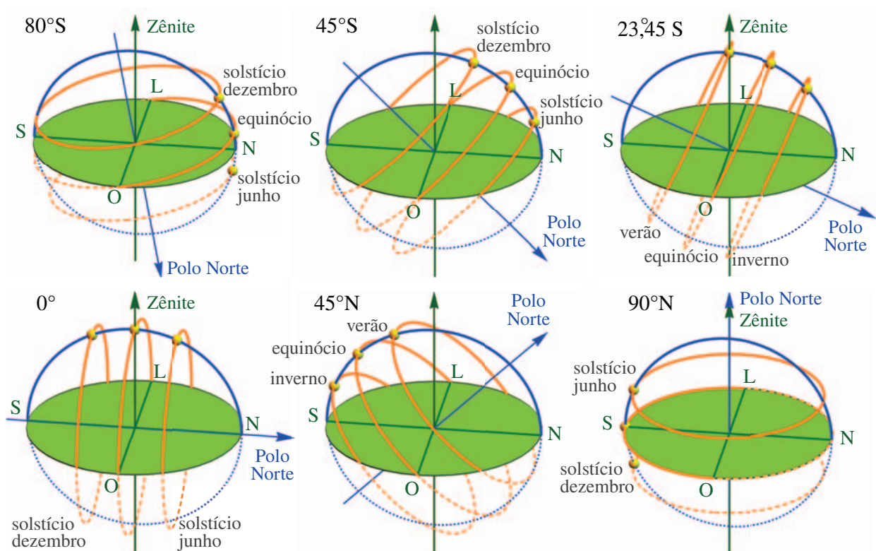
Figura 1.31: Trajetórias do Sol para observadores em diversas latitudes. As linhas laranjas representam em todos os painéis as trajetórias do Sol nos solstícios e equinócios (os dois equinócios correspondem à mesma linha). O disco verde (em perspectiva) representa o horizonte local. O círculo azul é o meridiano principal local (passa pelo Norte, Sul e zênite).
