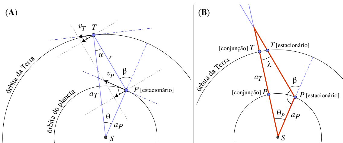
Figura 4.18: (A): Configuração planetária para determinarmos o momento em que um planeta interno ( P ) aparenta estar estacionário quando observado da Terra ( T ). v_T e v_P são as velocidades orbitais da Terra e do planeta, respectivamente, assumindo órbitas circulares de raios a_T e a_P . Suas projeções perpendiculares a linha \overline{PT} são iguais no ponto estacionário. (B): Configuração mostrando dois instantes, estacionário e em conjunção, para o cálculo do arco que o planeta executa em movimento aparente retrógrado.
