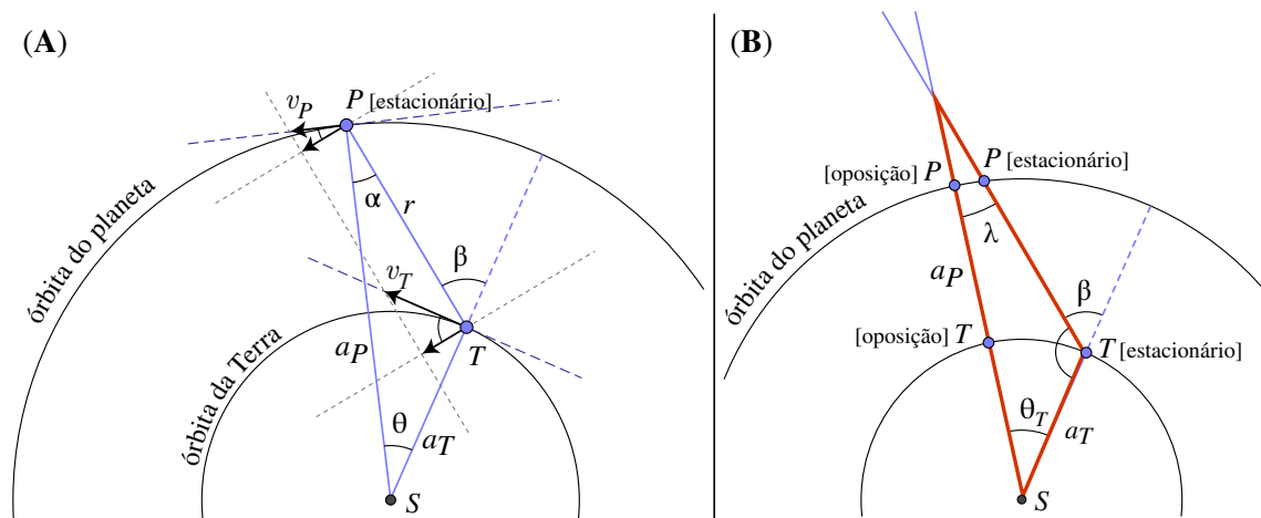
Figura 4.17: (A): Configuração planetária para determinarmos o momento em que um planeta externo ( P ) aparenta estar estacionário quando observado da Terra ( T ). v_T e v_P são as velocidades orbitais da Terra e do planeta, respectivamente, assumindo órbitas circulares de raios a_T e a_P . Suas projeções perpendiculares a linha \overline{PT} são iguais no ponto estacionário. (B): Configuração mostrando dois instantes, estacionário e em oposição, para o cálculo do arco que o planeta executa em movimento aparente retrógrado.
