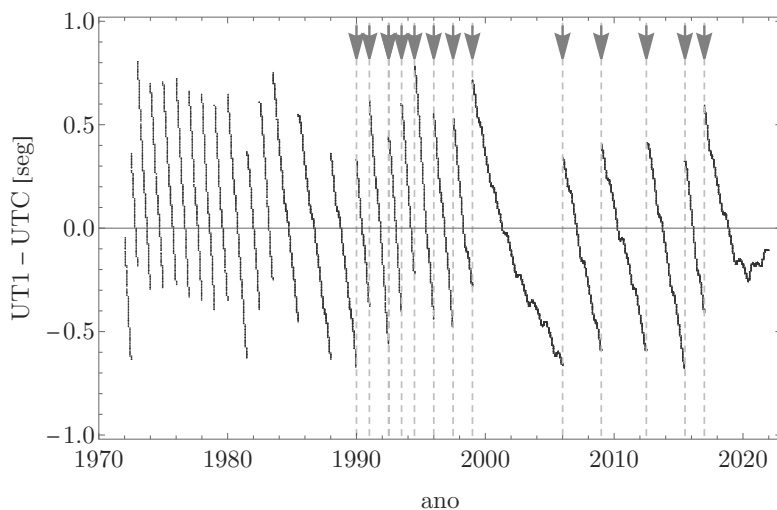
Figura 2.19: Diferença entre o UT1 e UTC em função do tempo. As discontinuidades correspondem à introdução de um segundo intercalar (as flechas indicam os últimos segundos intercalares). Figura feita com dados do IERS.
