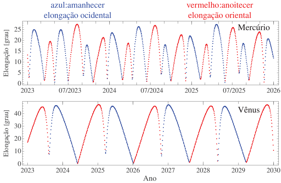
Figura 4.16: Variação da elongação dos planetas inferiores, Mercúrio e Vênus. A cor azul é quando o planeta é observado antes do Sol nascer e a cor vermelha indica quando o planeta é observado logo após o pôr do Sol. Note que a amplitude da elongação de Vênus é quase o dobro da de Mercúrio. Para Mercúrio, os pontos estão espaçados em intervalo de um dia; para Vênus de 3 dias. Note que a elongação muitas vezes não atinge 0^\circ , devido à inclinação relativa das órbitas com a eclíptica. Os dados foram obtidos com o Horizons System do JPL/NASA.
