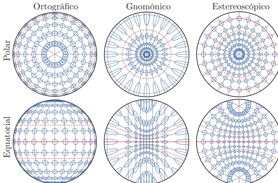
Figura 1.46: Indicatriz de Tissot (elipses/círculos azuis) para projeções azimutais, em aspectos polar e equatorial. As linhas de latitude (declinação) e longitude (ascensão reta) estão em intervalos de 15^\circ . O equador é a linha cheia vermelha. A projeção gnomônica é limitada em 76^\circ e a estereoscópica em 110^\circ para evitar deformações excessivas. A projeção ortográfica está limitada a 90^\circ por construção (a projeção ortográfica pode mostrar no máximo metade da esfera, isto é, um hemisfério).
