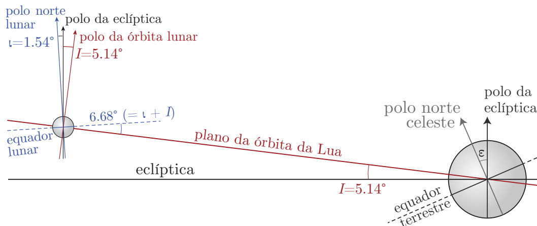
Figura 4.33: Configuração da Lua em sua órbita ao redor da Terra. O tamanho da Terra e da Lua estão em escala, mas as distâncias não estão. O ângulo de inclinação do equador lunar em relação à eclíptica (obliquidade da Lua) está fora de escala para facilitar a representação gráfica. A obliquidade da Terra é \varepsilon \simeq 23^{\circ},439 . Em relação ao equador terrestre, a órbita lunar tem uma inclinação de 28^{\circ},58 .
