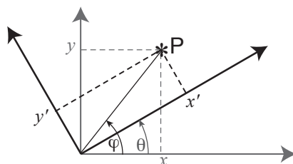
Figura 1.36: Rotação no plano de um ângulo \theta . As coordenadas do ponto P se escrevem como:
