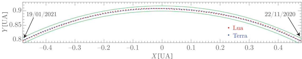
Figura 5.14: Trecho das trajetórias da Terra e da Lua ao redor do Sol entre novembro/2020 e janeiro/2021, observados de uma distância muito grande, perpendicular ao plano orbital (eclíptica) representados pelos eixos cartesianos X e Y em Unidades Astronômicas (UA). O baricentro do sistema Terra–Lua descreve uma elipse (linha cinza) ao redor do Sol [ou, mais precisamente, do centro de massa do Sistema Solar nas coordenadas (X, Y) = (0, 0) ] enquanto a Terra e a Lua oscilam em torno desta elipse. As linhas verdes representam a região de influência gravitacional da Terra (ver mais abaixo no texto). Olhando com atenção (e um bom zoom ), podemos ver as duas curvas no gráfico acima.
