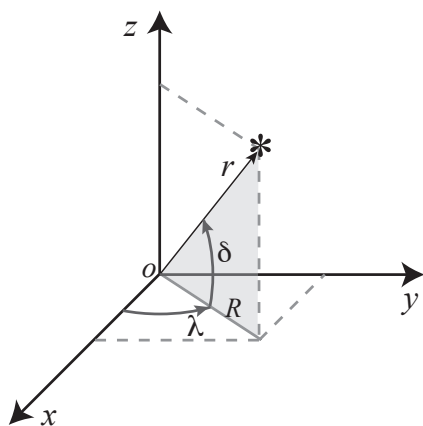
Figura 1.17: Coordenadas esféricas polares, \lambda e \delta de um ponto (sistema dextrogiro, isto é, \vec{x} \times \vec{y} = \vec{z} ). r é o raio vetor e R é a sua projeção no plano x - y . O ângulo longitudinal é medido a partir do eixo x no sentido anti-horário sobre o plano x - y .
