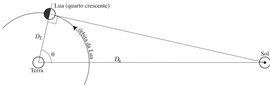
Figura 4.42: Método de Aristarco. D_L é a distância da Terra à Lua, D_\odot é a distância Terra–Sol. O ângulo \theta corresponde ao momento em que metade do disco lunar (visto da Terra) está iluminado (quarto crescente como na figura ou quarto minguante).
