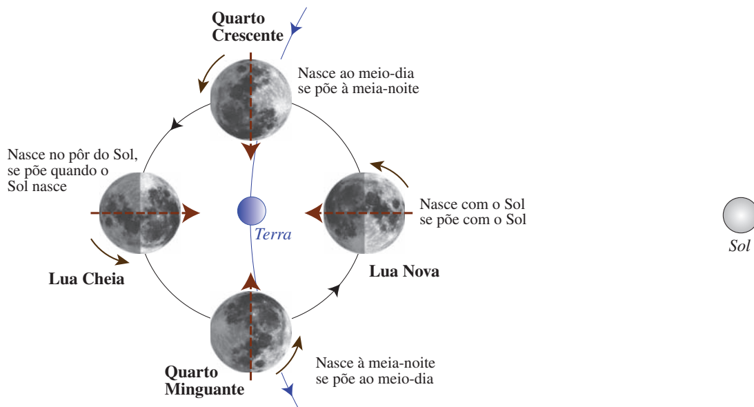
Figura 1.11: Movimento próprio da Lua em torno da Terra. Observe que a Lua apresenta sempre a mesma face voltada para Terra. A Lua gira em torno do seu próprio eixo com o mesmo período em que gira em torno da Terra (simbolizado pela flecha). Também vemos o momento em que a Lua em determinada fase nasce e se põe. Esta figura está completamente fora de escala; para o sistema Terra–Lua em escala realista veja a Fig. 4.38 na página 156.
