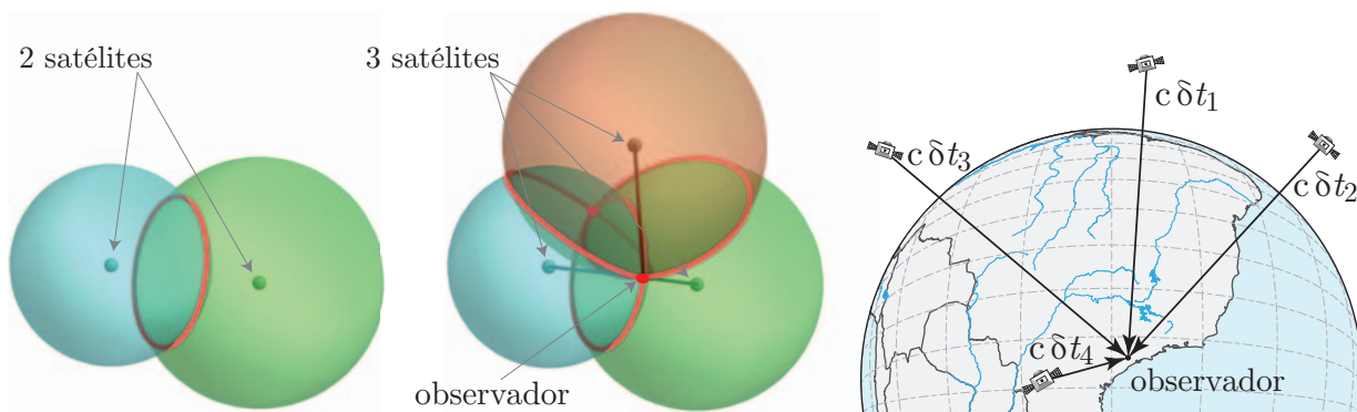
Figura 3.5: A intersecção de duas esfera é um círculo (em vermelho no painel a esquerda). A intersecção entre três esferas, se dá em 2 pontos. O usuário de um receptor GPS está em uma destas intersecções, captando o sinal de três satélites neste exemplo. O painel a direita mostra as pseudo-distâncias c\delta t_i de cada um dos 4 satélites necessários para determinar a posição do observador, onde \delta t é o intervalo de tempo que o sinal leva para chegar no receptor.
