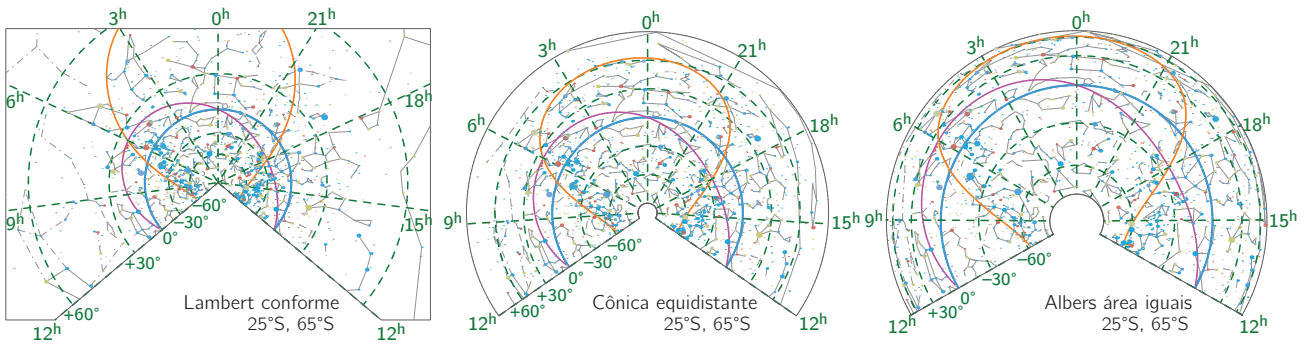
Figura 1.44: Comparação de três projeções cônicas: Lambert (conforme), Cônica equidistante e Albers (áreas iguais). Todas mostram a mesma região da esfera celeste em coordenadas equatoriais centradas no Polo Sul, com paralelos padrões 25 S e 65 S. O equador celeste é a linha em ciano, em magenta está representada a eclíptica e o equador galáctico em cor laranja.
