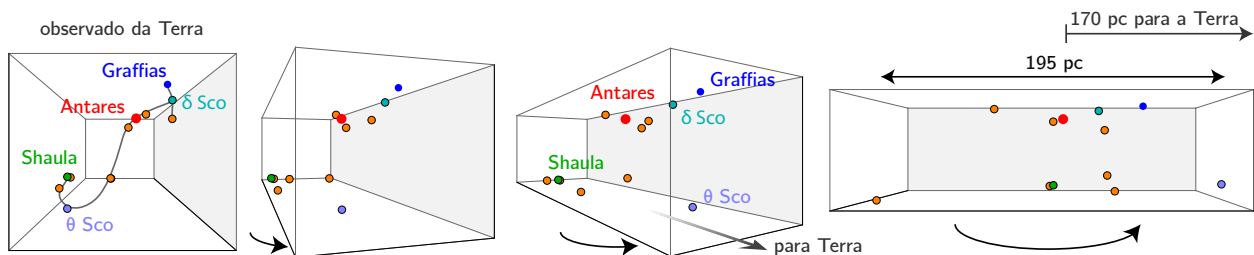
Figura 1.6: Exemplo da mudança da posição aparente (projetada) das estrelas da constelação do Escorpião. À esquerda, o padrão observado da Terra e à direita as mesmas estrelas vistas por um observador hipotético. Parsec (pc) é uma unidade de distância que equivale a 3,26 anos-luz (a definição será dada na seção 3.7.1).
