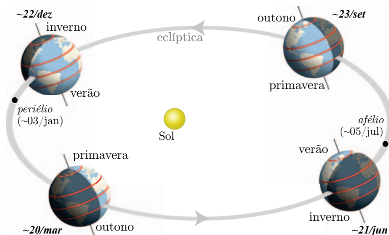
Figura 1.24: As estações do ano ocorrem devido à inclinação do eixo da Terra em relação ao seu plano orbital ao redor do Sol, e nada tem a ver com a distância da Terra ao Sol. Os círculos vermelhos sobre a Terra representam o equador, os trópicos e os círculos polares. Na figura, a órbita parece mais achatada para criar um efeito de perspectiva.
