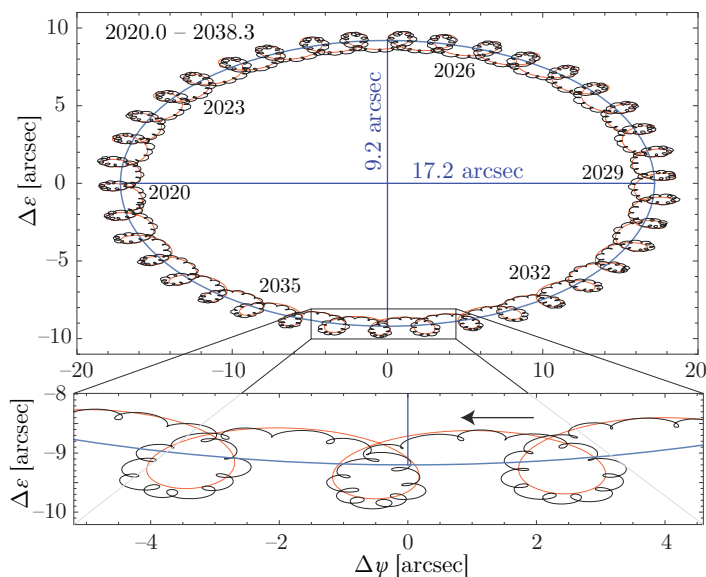
Figura 3.14: Variação da obliquidade ( \Delta\epsilon ) e longitude ( \Delta\psi ) devido à nutação. A elipse azul representa o principal termo da nutação de 18,61 anos, com os semi-eixos indicados. A linha laranja mostra o efeito de usarmos também o 2º termo de 164,9 dias da nutação. Em destaque, abaixo, detalhe do movimento de nutação calculado com o modelo IAU2000A.
