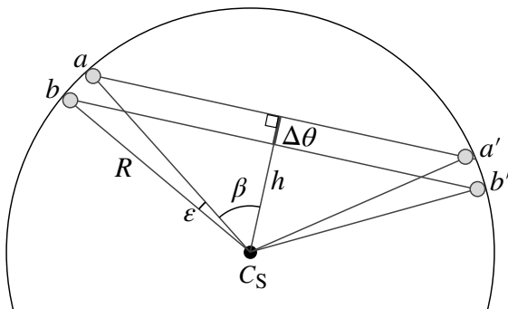
Figura 4.47: Geometria dos trajetos aparentes de Vênus (fora de escala) sobre o disco solar, observado em duas latitudes diferentes (linha \overline{aa'} e \overline{bb'} ). C_s é o centro do disco solar.
