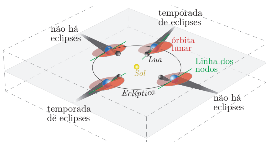
Figura 4.29: Duas vezes por ano (excepcionalmente até 3 vezes) a Lua, Terra e Sol estão alinhados próximos da linha dos nodos: nestes casos temos as temporadas de eclipses. Quando a conjunção não está alinhada com a linha dos nodos, a sombra da Lua não atinge a Terra e nem a Lua passa pela sombra da Terra.
