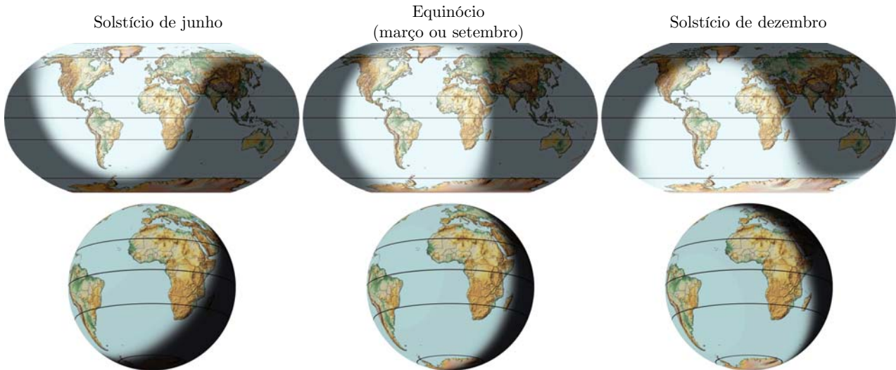
Figura 1.27: Iluminação da Terra no início das estações do ano (solstícios e equinócios) ao meio-dia de Brasília (exceto para o solstício de dezembro, quando o horário de verão pode estar em vigência em alguns estados). Na linha de cima vemos os planisférios com projeção Robinson (linhas de latitudes paralelas) e abaixo na forma de um globo (projeção ortográfica).
