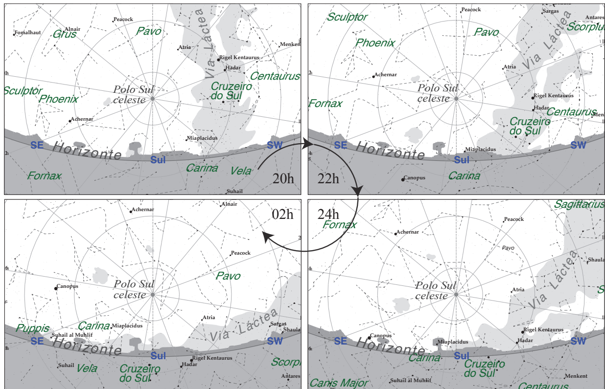
Figura 1.8: Polo celeste sul visto de São Paulo no início de setembro em 4 instantes diferentes: às 20, 22, 24, e 2 horas. Os círculos representam as Declinações e as retas são as Ascensões Retas (este sistema de coordenadas será definido na seção 1.5.2). O tamanho das estrelas é proporcional ao brilho aparente. Estando no Hemisfério Sul e olhando para a direção sul, veremos os astros girando em torno do Polo Sul Celeste no sentido horário . No Hemisfério Norte, veríamos os astros girando em torno do Polo Norte Celeste no sentido anti-horário .
