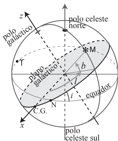
Figura 1.23: Sistema de coordenadas galácticas. O astro M tem coordenadas longitude galáctica ( l ) e latitude ( b ). O ponto N é a intersecção do plano galáctico com o equador celeste (o nodo), C.G. é a direção do centro da Galáxia (que fica na constelação de Sagitário) e i é a inclinação do plano galáctico em relação ao equador celeste.
