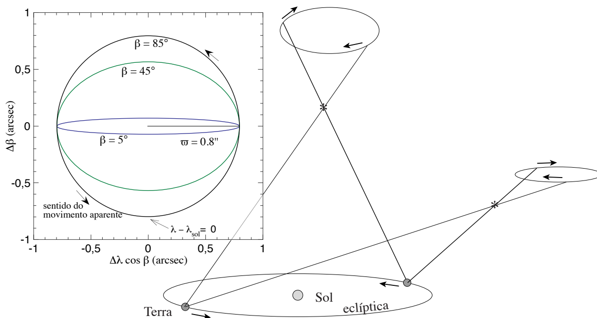
Figura 3.23: Elipse paraláctica. Trajetória aparente devido ao efeito de paralaxe anual. O gráfico a esquerda ilustra um exemplo com \varpi = 0{,}8'' e diferentes latitudes. Quando o astro se encontra no polo da eclíptica, sua trajetória aparente é praticamente um círculo; quando o astro está na eclíptica ( \beta = 0 ) sua trajetória é um “vai-e-vem” linear.
