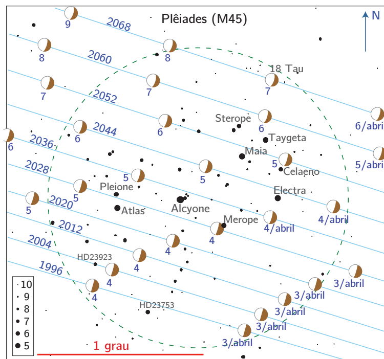
Figura 4.20: Trânsito de Vênus pelas Plêiades, que ocorrem aproximadamente a cada 8 anos e duras alguns dias. As linhas diagonais em azul indicam a trajetória de Vênus visto da Terra com o ano indicado. Os números próximos da primeira imagem de Vênus de cada linha correspondem ao dia em abril às 0h UT. O círculo tracejado representa aproximadamente a região onde se encontram as Plêiades. Embaixo, a esquerda, está a escala de magnitude das estrelas.
