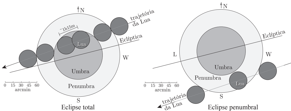
Figura 4.27: Esquerda: Exemplo de um eclipse da Lua visto da Terra (a umbra e a penumbra não são realmente visíveis). Neste exemplo a totalidade (intervalo de tempo em que a lua permanece na umbra terrestre) dura cerca de 1 hora e 15 minutos. Direita: Exemplo de um eclipse da Lua penumbral, quando a Lua não passa pela umbra da Terra.
