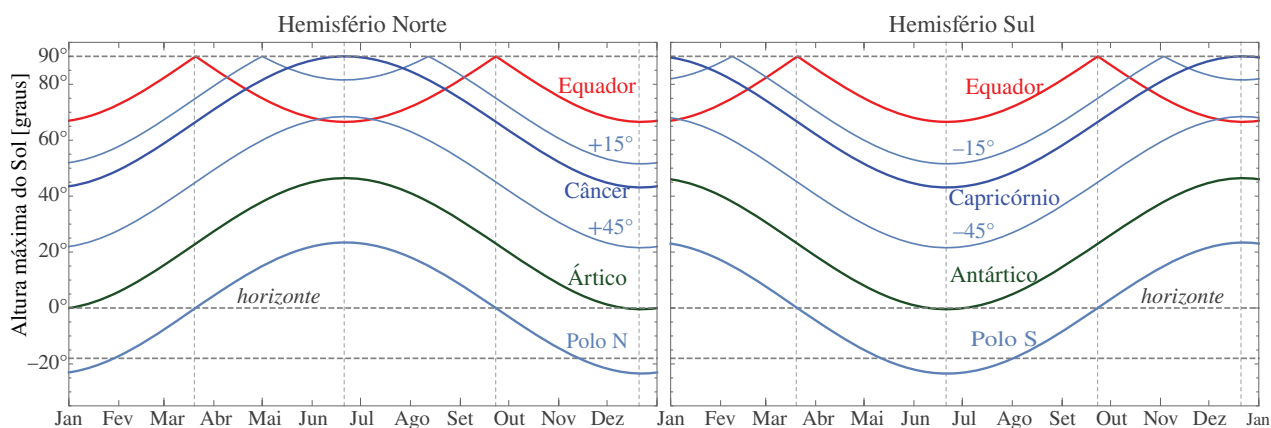
Figura 1.33: Variação da altura máxima do Sol ao longo do ano para diversas latitudes. As linhas verticais indicam os equinócios e solstícios. As linhas horizontais mostram a altura máxima ( 90^{\circ} , isto é, o zênite), o horizonte ( 0^{\circ} ) e a altura abaixo da qual a noite é completamente escura ( -18^{\circ} ). Esta figura pode ser comparada com a Fig. 1.31, que mostra a trajetória aparente diurna do Sol para observadores em várias latitudes.
