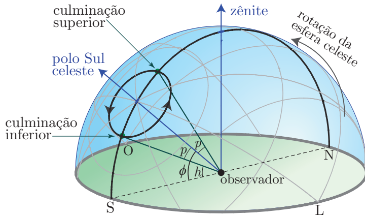
Figura 1.32: Altura de um astro circumpolar observado no Hemisfério Sul nos momentos de culminação superior e inferior devido ao movimento aparente diário. O ângulo \phi é a altura do polo celeste e a latitude do observador e o ângulo p é medido entre os pontos de culminação superior e inferior em relação ao polo celeste. A altura da culminação inferior neste exemplo é h . Se p for maior que a distância zenital do polo celeste, a culminação superior se dá na direção oposta do polo em relação ao zênite.
