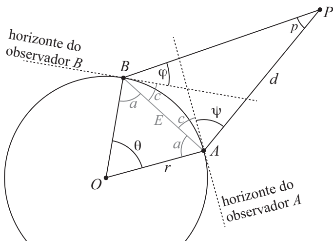
Figura 4.41: Geometria para determinação da distância topocêntrica d entre o observador A e o objeto P , com auxílio da observação de B .
