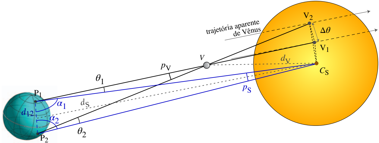
Figura 4.45: Observação do trânsito de Vênus (V) pelos observadores P_1 e P_2 (em latitudes diferentes e não necessariamente na mesma longitude). O disco de Vênus observado por P_1 e P_2 está representado por V_1 e V_2 , respectivamente. A distância entre as trajetórias aparentes é \Delta\theta (note que é uma distância angular observada). Os ângulos p_V e p_S são as paralaxes de Vênus e do Sol, respectivamente. C_S é o centro do Sol. A distância d_{12} entre os observadores é uma reta que passa pelo interior da Terra.
