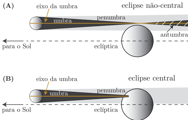
Figura 4.21: Configuração geométrica de um eclipse não-central (Painel (A), acima), quando o eixo da umbra não toca na Terra e configuração de um eclipse central (Painel (B), abaixo). A linha tracejada indica o plano orbital da Terra ao redor do Sol, a eclíptica. O Sol está à esquerda, distante, indicado pela seta.
