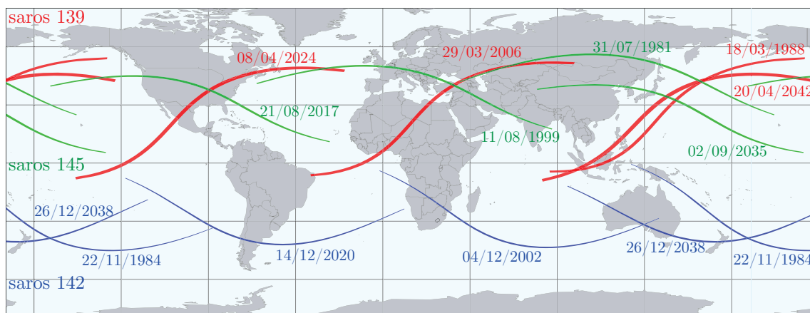
Figura 4.31: Exemplo da semelhança da geometria de eclipses da mesma série de saros (aqui, series 139 [vermelho], 142 [azul] e 145 [verde]). A cada 18 anos, 11 dias e 8 horas, os eclipses se repetem a 120^\circ para o Oeste (o que corresponde a 8h) de forma muito semelhante. A cada 3 saros, alguns eclipses praticamente ocorrem da mesma forma e no mesmo local (por exemplo, na serie de saros 139 de 1988 e 2042).
