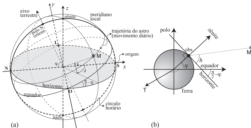
Figura 1.18: Sistema de coordenadas horizontal. O astro M tem coordenadas h (altura) e A (azimute). Os “polos” deste sistema são o zênite e o nadir. O azimute é medido a partir do Sul em direção ao Oeste, ao longo do horizonte (o círculo principal neste sistema). A altura é positiva em direção ao zênite e negativa em direção ao nadir. Também são mostrados na figura os eixos cartesianos x , y e z .
