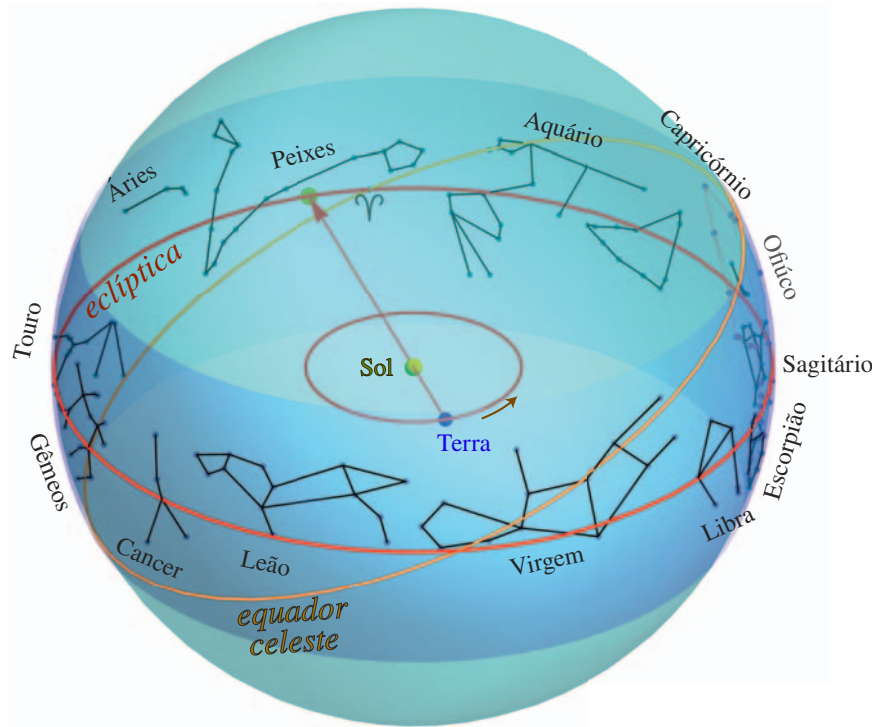
Figura 1.5: O movimento aparente do Sol visto da Terra (círculo no final da flecha) durante um ano, percorrendo as constelações do Zodíaco. A constelação de Ofiúco está no caminho do Sol, mas não é considerada uma das 12 constelações do Zodíaco. As linhas da eclíptica e equador celeste serão definidas mais a frente. O símbolo ♈ representa o ponto vernal na intersecção da eclíptica com o equador celeste.
