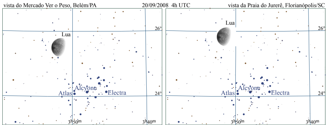
Figura 4.40: Paralaxe da Lua. A Lua e as Plêiades observadas simultaneamente em dois lugares com a mesma longitude, mas latitudes diferentes. Note a diferença da posição da Lua. A diferença em latitude é de cerca de 26 graus (ou 2872 km).
