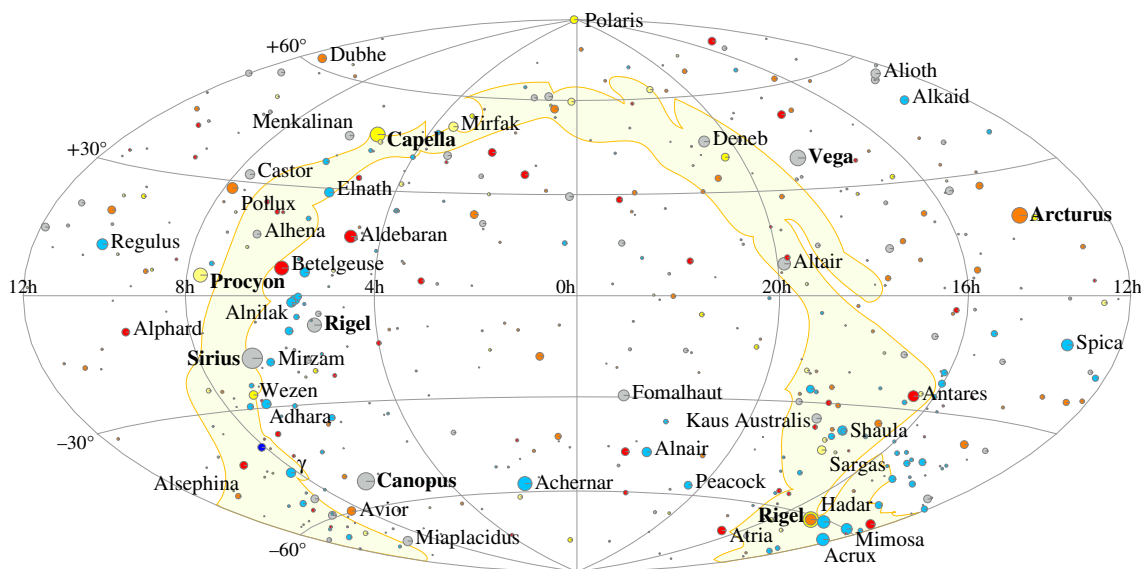
Figura 1.20: Planisfério em coordenadas equatoriais usando projeção Aitoff. O centro do planisfério é o ponto vernal, ♈. A estrela Polaris se encontra praticamente no polo celeste Norte. As estrelas mais brilhantes também estão listadas na Tabela 1.2.
