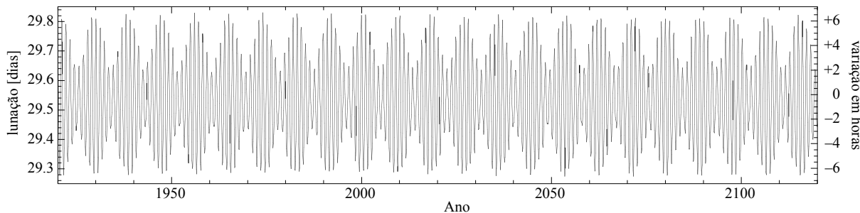
Figura 2.10: Duração de uma luação (mês sinódico, período entre duas luas novas) em um período de 200 anos. No eixo à direita é mostrada a variação em horas em relação ao período médio de luação.
