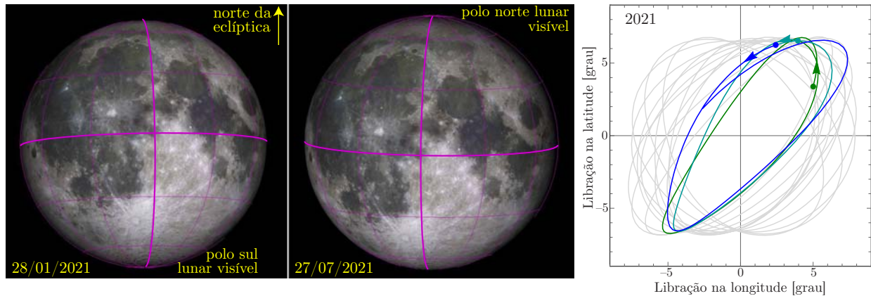
Figura 4.34: Esquerda e centro: Exemplo da libração da lua, tanto em longitude como em latitude com imagens da Lua. Note a mudança das posições das crateras e “mares” próximos da borda da Lua. Os traços em magenta representam as coordenadas selenográficas . Direita: movimento relativo da coordenada selenográfica ( 0^\circ , 0^\circ ) mostrando a libração. O traço verde corresponde a janeiro/2021, o ciano a fevereiro e o azul a março. Em cinza claro, o restante do ano de 2021. Os círculos representam o início de cada mês e a flecha indica a direção do movimento de libração.
