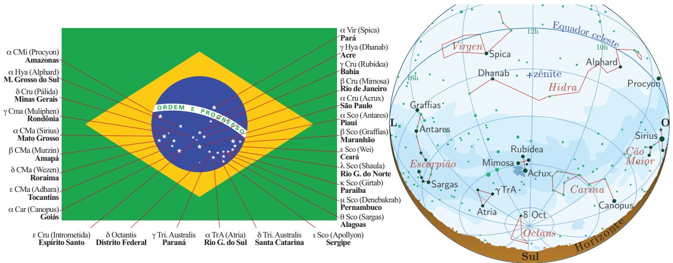
Figura 1.7: Esquerda: Bandeira oficial do Brasil com a identificação das estrelas e estados. Direita: Representação da esfera celeste que seria observada em 15/11/1889 às 8h30 no RJ (as estrelas da bandeira estão em destaque, mais escuras e maiores). Note que o “céu” da bandeira está invertido em relação ao céu que observamos da Terra.
