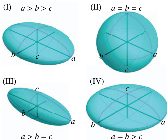
Figura 3.1: Exemplo de elipsoides. (I) Elipsoide triaxial (3 eixos diferentes); (II) Esfera (3 eixos iguais); (III) Elipsoide prolato (2 eixos iguais menores que o eixo maior); (IV) Elipsoide oblato (2 eixos iguais, maiores que o eixo menor). O elipsoide que representa a Terra é aproximadamente oblato (mas não tão exagerado quando esta figura).
