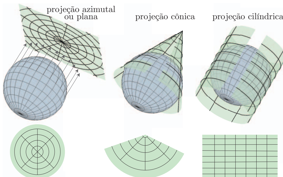
Figura 1.42: Tipo de projeções usadas em planisférios. Cada ponto da superfície da esfera corresponde a um ponto da superfície plana (projeção azimutal, caso polar), cônica ou cilíndrica dada pelas Eqs. (1.36). Lembramos que tanto o cone quanto o cilindro podem ser “desenrolados” sem deformação e são, portanto, equivalentes ao plano.
