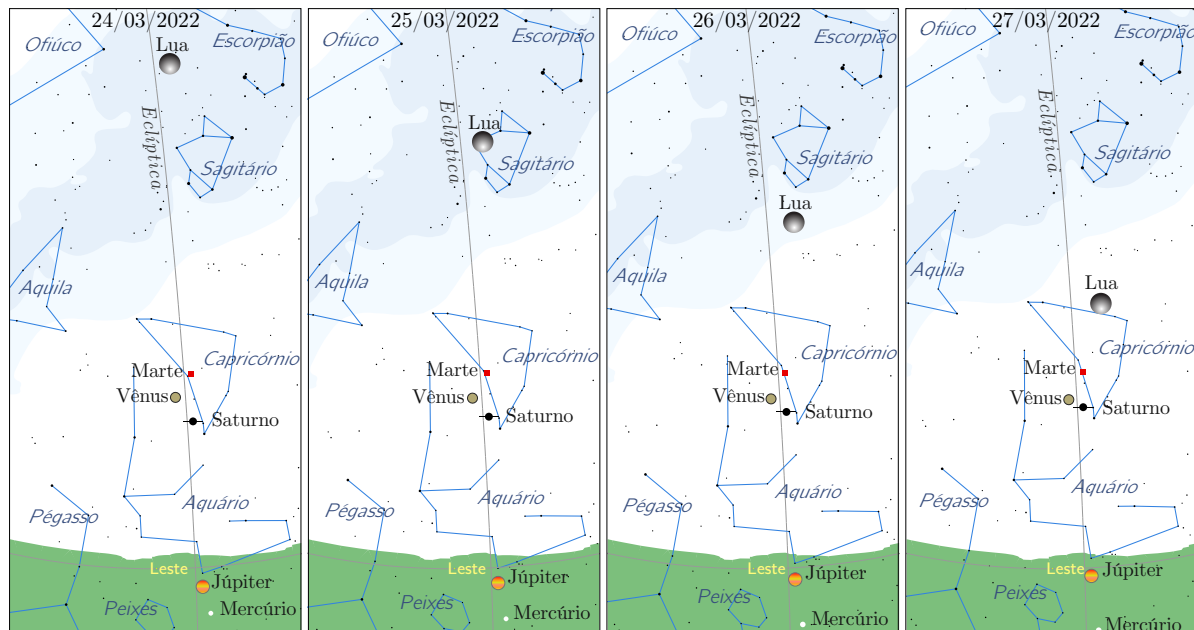
Figura 1.10: Movimentos aparentes na esfera celeste. O movimento aparente da Lua em relação às estrelas fixas pode ser notado comparando as imagens de observações em São Paulo em dias consecutivos feitas no mesmo horário (5h da manhã, hora local). A região verde representa o horizonte na direção Leste e as regiões cinzas representam a Via Láctea. Observe também que as estrelas também apresentam um movimento; a cada dia as estrelas se levantam (“nascem”) cerca de 4 minutos mais cedo. Também podemos notar o movimento aparente de Vênus e Mercúrio (abaixo do horizonte, portanto não observável na realidade) em relação às estrelas “fixas”. Já o movimento próprio de Júpiter e Saturno são imperceptíveis em apenas 4 dias na escala desta figura.
