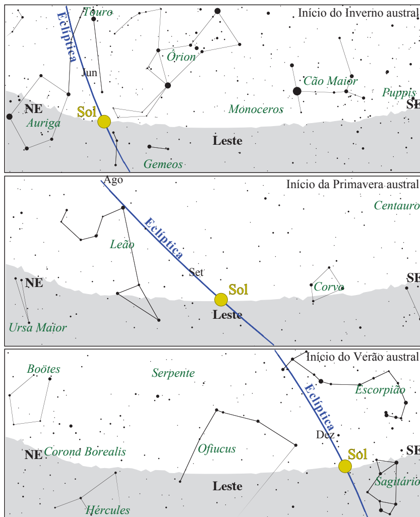
Figura 1.13: Variação anual da trajetória aparente do Sol durante o ano (p. ex., para um observador em São Paulo). No início do Inverno do Hemisfério Sul, o Sol “nasce” na direção do Nordeste; no início da primavera, na direção Leste; e no início do Verão austral, na direção Sudeste.
