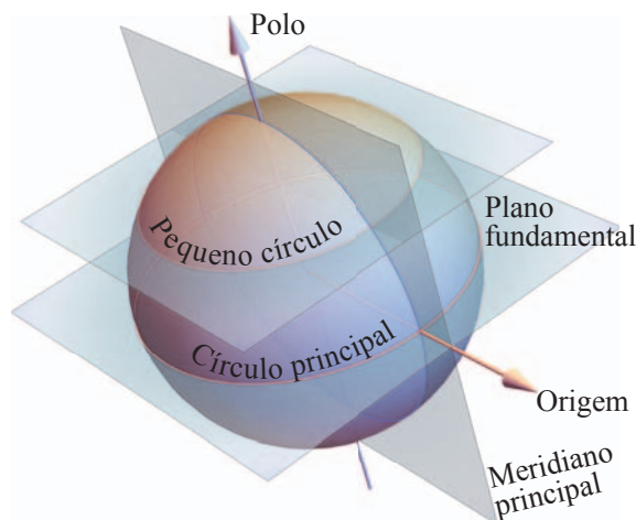
Figura 1.16: As coordenadas em uma esfera são definidas através de um plano fundamental que corta a esfera em duas metades, passando pelo centro (definindo um círculo principal ou equador) e um ponto arbitrário no equador. Através deste ponto traça-se um outro grande círculo, perpendicular ao “equador”, definindo-se assim o meridiano principal. Planos que cortam a esfera, mas não passam pelo centro, definem os pequenos círculos.
