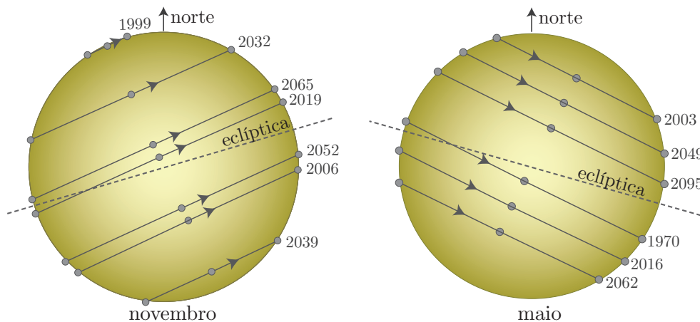
Figura 4.19: Trânsitos de Mercúrio vistos da Terra no nodo ascendente (novembro) e no nodo descendente (maio). Note a simetria dos trânsitos, alternando entre o norte e sul em relação à eclíptica. O trânsito de novembro/1999 foi de raspão.
