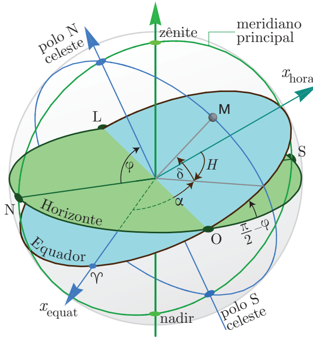
Figura 1.21: Sistema de coordenadas horárias. O astro M tem coordenadas ângulo horário ( H ) e declinação ( \delta ). A ascensão reta, \alpha , também é medida ao longo do equador celeste, porém a partir do ponto vernal. A latitude do observador é \varphi , portanto o ângulo entre o equador celeste e o horizonte é \pi/2 - \varphi . Os eixos x_{\text{hora}} e x_{\text{equat}} correspondem aos sistemas horário e equatorial, respectivamente. Como o polo Norte celeste está acima do horizonte, este exemplo é de um observador do Hemisfério Norte.
