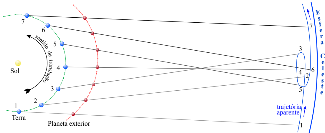
Figura 1.15: Posições da Terra e Marte em suas órbitas em torno do Sol no mesmo período do Fig. 1.14. Entre as posições marcadas 1 e 3, o movimento aparente de Marte é direto. Entre as posições 3 e 5 (quando o planeta está estacionário), o movimento é retrógrado e, em seguida volta a ser direto. Em 4, Marte está em oposição (isto é, o Sol, a Terra e Marte estão aproximadamente alinhados). As posições nas órbitas correspondem a intervalos de 4 semanas.
