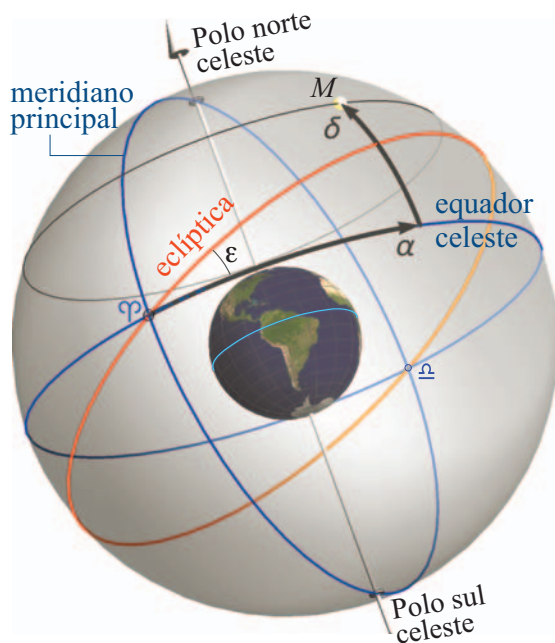
Figura 1.19: Sistema de coordenadas equatoriais. O astro M tem coordenadas ascensão reta ( \alpha , medida a partir do ponto vernal, \gamma ) e declinação ( \delta ). Atualmente, a inclinação do equador celeste em relação à eclíptica, \varepsilon , é de aproximadamente 23^{\circ}26'21'',45 no início do ano 2000.
