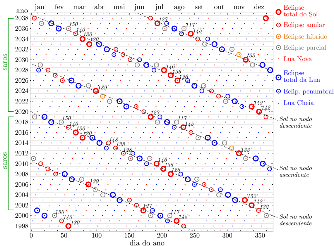
Figura 4.30: Frequência dos eclipses solares e lunares. Os eclipses se agrupam em diagonais correspondendo aos eclipses que ocorrem no nodo ascendente ou descendente da órbita lunar. Os grupos de 2 ou 3 eclipses que ocorrem no intervalo de cerca de 34 dias correspondem às “temporadas de eclipses”. O período de saros (ou simplesmente saros) tem um pouco mais de 18 anos e a figura ilustra 2 exemplos. Alguns eclipses têm o número de sua série de saros destacadas.
