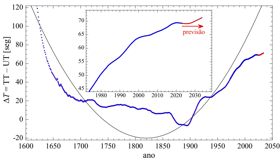
Figura 2.12: \Delta T = TT - UT (ou, antigamente, ET - UT , como será visto mais abaixo) em segundos. Os valores para os anos superiores a 2023 são previsões (pontos vermelhos) cujas incertezas são de cerca de 1 segundo para o ano 2023 e \sim 5 segundos para 2033. A parábola (linha contínua em cinza) representa o comportamento secular esperado quando consideramos vários séculos para o passado ou futuro. Fonte: IERS Rapid Service/Prediction Center
