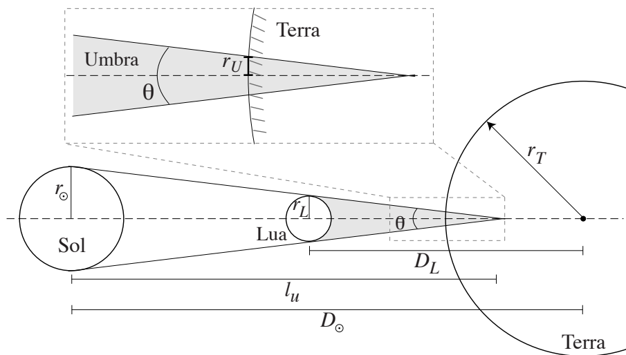
Figura 4.25: Geometria de um eclipse do Sol para estimarmos o tamanho da umbra na superfície terrestre.
