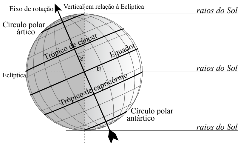
Figura 1.26: Diagrama ilustrando a definição dos trópicos de câncer e capricórnio e os círculos polares. O ângulo \varepsilon é a inclinação do eixo da Terra (obliquidade da eclíptica). Como o Sol está muito distante, podemos assumir que os raios de luz chegam paralelos na Terra. A figura corresponde ao momento do solstício no Hemisfério Sul. Após seis meses, os raios do Sol chegam perpendicularmente no Trópico de Câncer (solstício do Hemisfério Norte).
