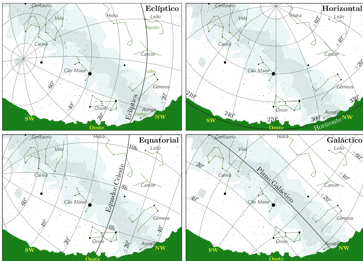
Figura 1.34: Exemplo de quatro sistemas de coordenadas, para um observador em São Paulo no início do Outono, por volta das 22h, olhando para a direção Oeste. A região em cinza escuro representa o horizonte geográfico local, em cinza claro a Via Láctea e a Grande Nuvem de Magalhães (próxima do polo Sul da eclíptica). Em cada um dos painéis podemos ver o círculo principal do sistema de coordenadas.
