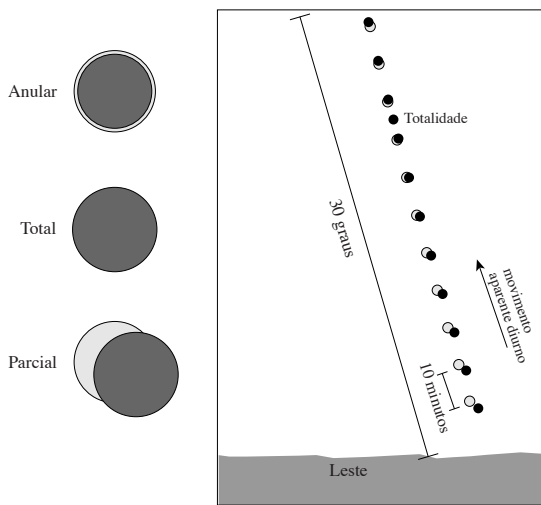
Figura 4.24: A esquerda, os três tipos de eclipse do Sol. No caso do eclipse anular, a Lua se encontra próxima do apogeu e seu diâmetro aparente é menor do que o do Sol; no eclipse total, a Lua se encontra próxima do perigeu. A direita, representação da observação de um eclipse do Sol.
