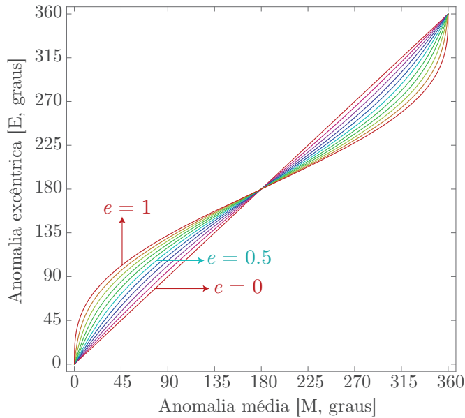
Figura 5.13: Relação entre as anomalias médias, M , e excêntrica, E , para excêntridades de zero a um (em passos de \Delta e = 0,1 ) obtidas pela solução numérica da equação de Kepler.
