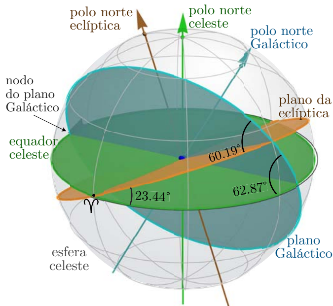
Figura 1.35: Posições relativas dos 3 principais planos de referência celestes, Equatorial, Eclíptica e Galáctico. Também estão ilustrados os eixos perpendiculares aos planos fundamentais e os ângulos de intersecção entre eles. Também está indicado o ângulo do nodo do plano Galáctico, medido a partir do ponto vernal, \Upsilon . Os ângulos são válidos para J2000 e variam lentamente com o tempo.
