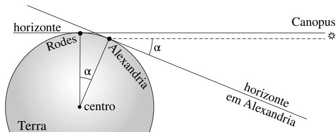
Figura 4.7: Método de Posidônio para determinar a circunferência da Terra. A estrela Canopus é observada na altura do horizonte em Rodas, mas atinge uma altura \alpha acima do horizonte de Alexandria. Este ângulo \alpha corresponde à diferença em latitude das duas cidades.
