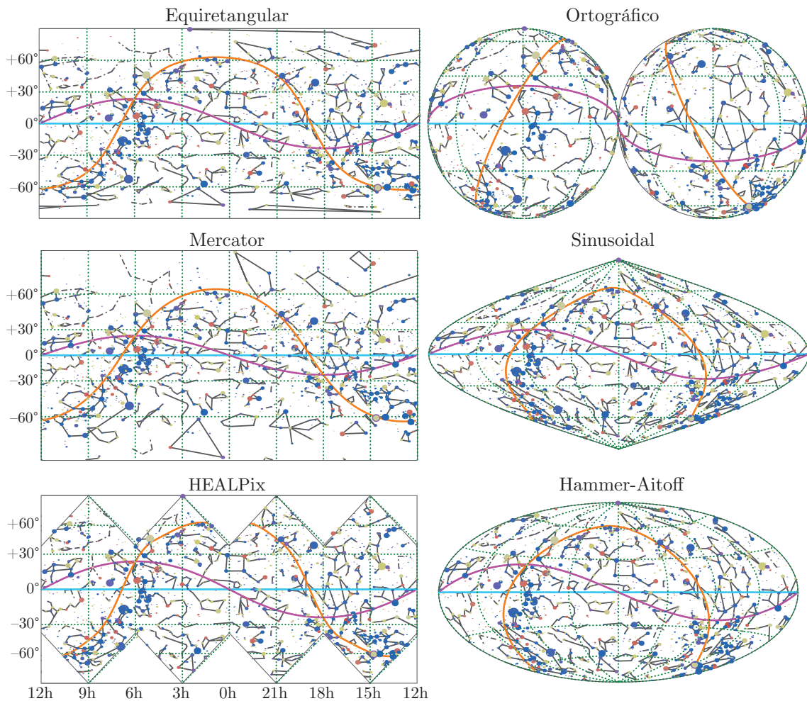
Figura 1.45: Exemplos de projeções de toda a esfera. O sistema de coordenadas é o equatorial (a linha ciano horizontal representa o equador celeste). Também estão representados a eclíptica (magenta) e o plano Galáctico (plano da Via Láctea em laranja). As estrelas mais brilhantes são mostradas junto com as linhas simbólicas das constelações.
