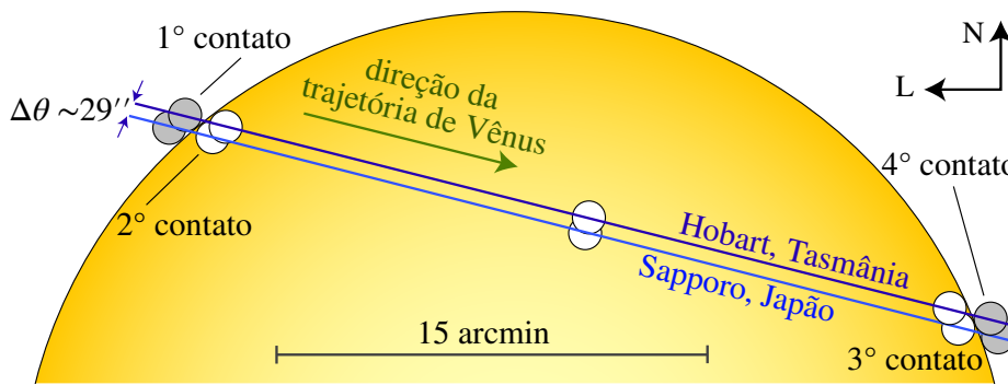
Figura 4.46: Trânsito de Vênus de 05/06/2012 observado de Sapporo, Japão e Hobart, Tasmânia. Os tamanhos dos discos de Vênus e do Sol estão em escala, assim como as trajetórias. No Japão, o trânsito de Vênus foi mais longo e de maior duração comparado ao trânsito observado na Tasmânia.
