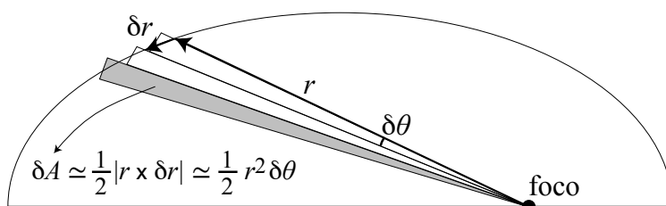
Figura 5.9: Área varrida pelo raio vetor r que percorre uma elipse. O ângulo \delta\theta subtende o segmento \delta r .
