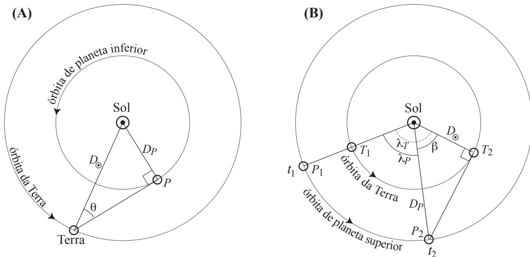
Figura 4.43: Método de Copérnico para determinação da distância dos planetas ao Sol. (A) Geometria para os planetas inferiores (ou interiores); (B) geometria para os planetas superiores (ou exteriores). Para os planetas superiores são necessárias duas medidas em dois momentos distintos, t_1 e t_2 .
