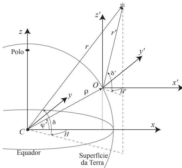
Figura 3.25: Efeito da paralaxe diária na posição de um astro próximo devido à rotação da Terra. Observando-se um astro próximo com 12 horas de intervalo, a posição aparente desta se desloca em relação ao fundo de estrelas distantes. O ângulo p é a paralaxe do astro, r é a distância geocêntrica e r' a distância topocêntrica.
