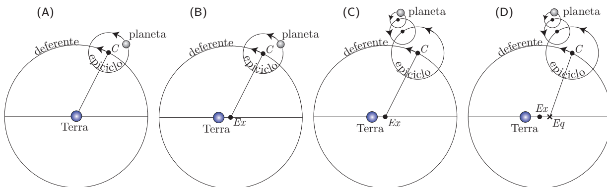
Figura 4.8: Sistema de epiciclos. (A): a Terra se encontra no centro do círculo (deferente) onde o epiciclo orbita. O planeta por sua vez gira em torno do ponto C , centro do epiciclo. (B): Hiparco notou que, para levar em conta a velocidade variável no movimento anual do Sol, a Terra deveria ser deslocada do centro do deferente ( Ex ). Isto é, existe uma excentricidade na posição da Terra (ainda hoje se emprega este termo quando nos referimos a elipses, cujo centro não coincide com o foco). (C): Para poder explicar precisamente todas as irregularidades das órbitas dos planetas, Hiparco introduziu epiciclos que giram em torno de epiciclos. (D) Ptolomeu introduziu o equante ( Eq , indicado por um “X”); para um observador hipotético no equante, o centro do epiciclo se move com velocidade constante ao longo do deferente.
