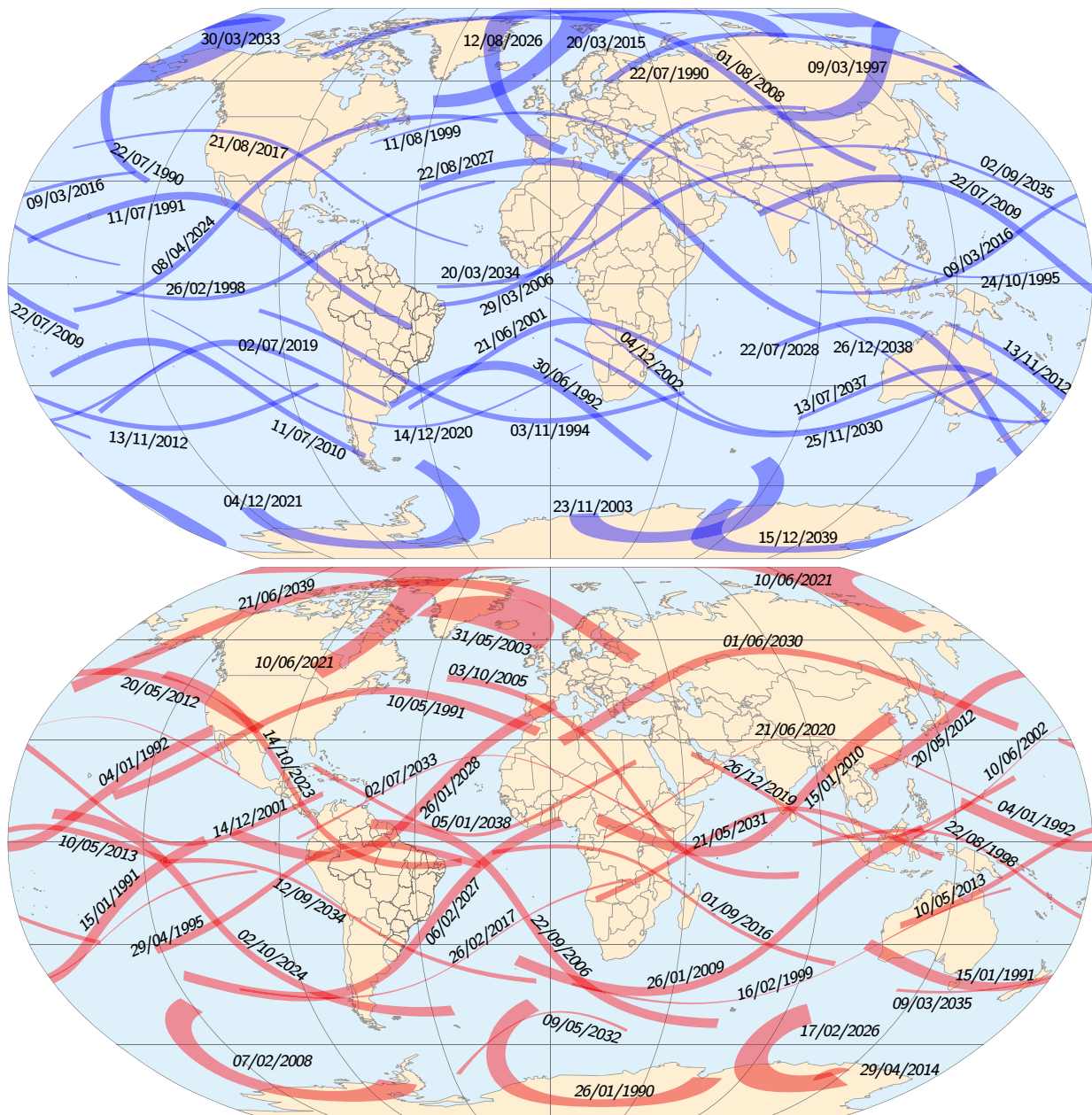
Figura 4.32: Eclipses do Sol (acima em azul os totais e abaixo em vermelho os anulares) entre 1990 e 2040. A trajetória da sombra da Lua na superfície da Terra se movimenta de Leste a Oeste. Os cálculos das trajetórias dos eclipses foram feitos por Fred Espenak, NASA/Goddard Space Flight Center. A projeção usada aqui é de Robinson. Para mais informações, veja o site : http://eclipsewise.com/ .
