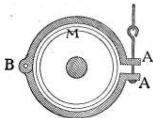
Esquema núm. 43 — Freno exterior
