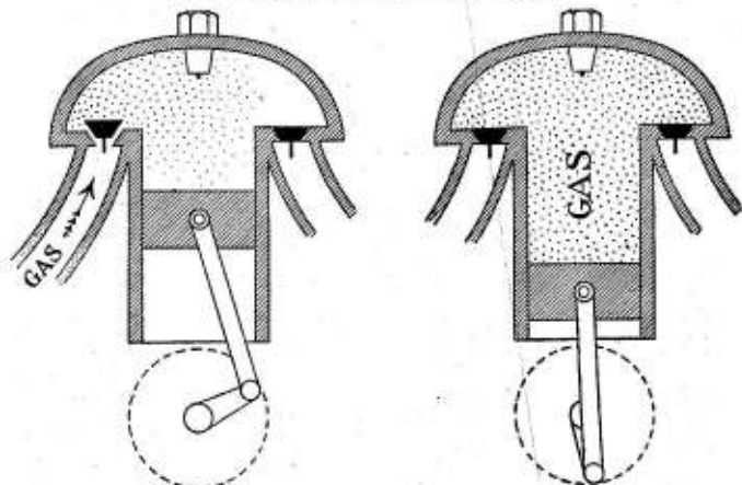
Esquema núm. 8. — El cilindro aspira el gas. La válvula de admisión está abierta y la de escape cerrada (Admisión)
