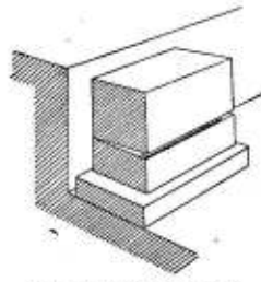
Solo un rodillo puesto a un lado sostiene el bloque. Lo restante de la mole queda en reposo
