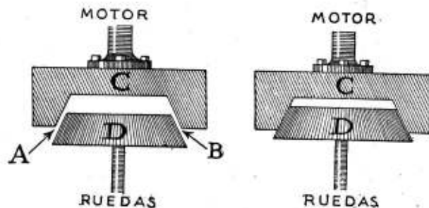
Esquema núm. 23. — A la izquierda el mecanismo está «desembragado», y a la derecha embragado, o sea para marchar el automóvil
