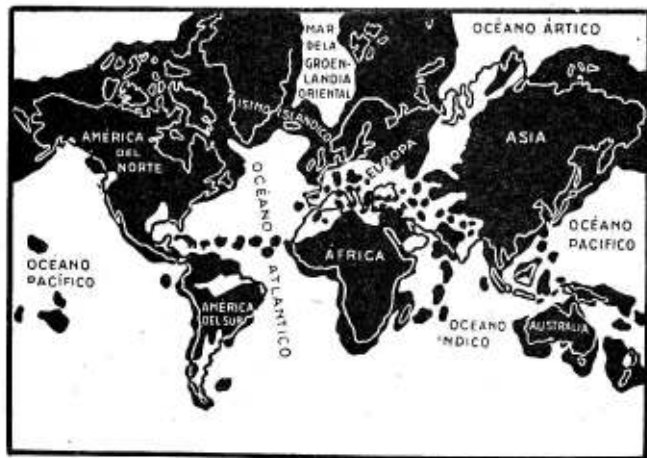
Continents y mares durante la era terciaria
